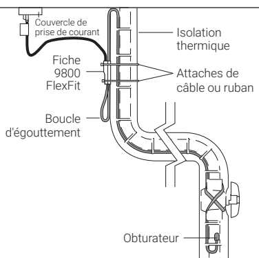
Figure 1. Installation type d'habitation préfabriquée
