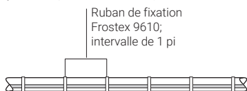
Figure 3. Méthode une passe
